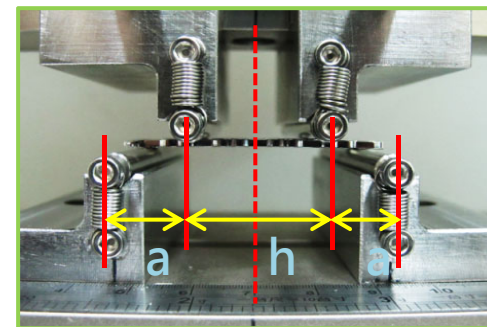
實驗架設圖
