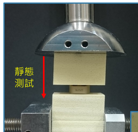
實驗架設圖
