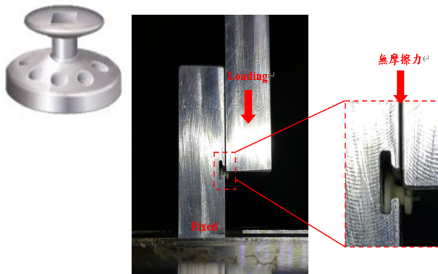
舌側扣剪力測試
