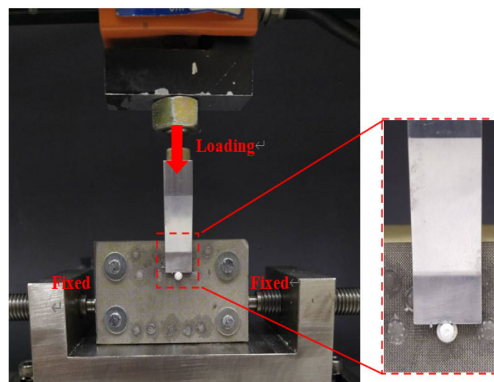
舌側扣抗剝離測試
