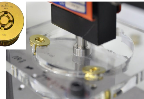
顱骨固定夾力學測試
