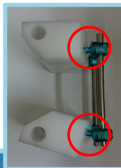
疲勞後滑移
