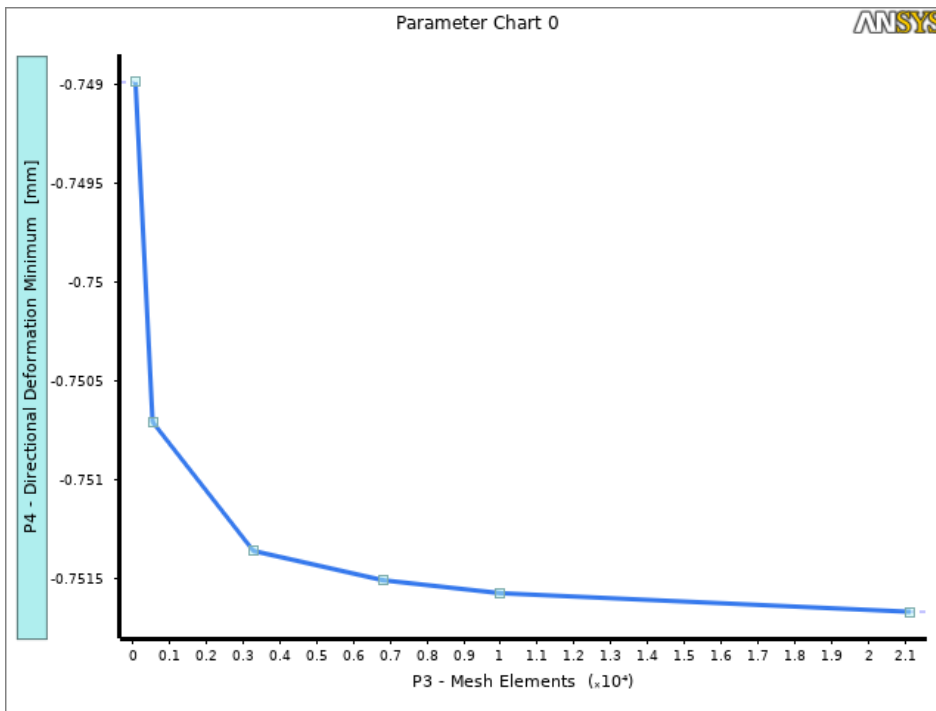
Tet mesh
