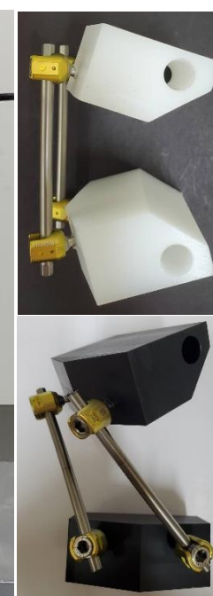
ASTM F1717-椎弓螺釘
